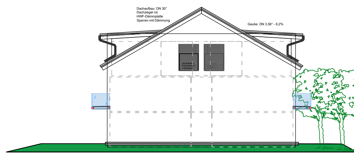
ANSICHT LINKS
