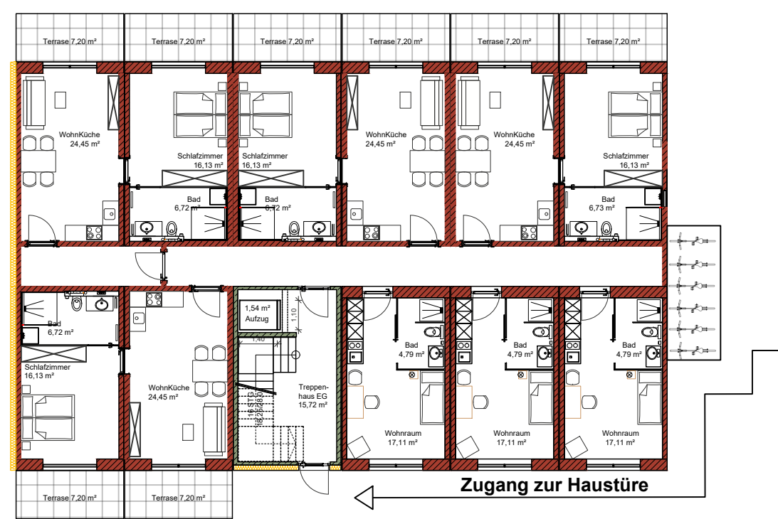
GRUNDRISS ERDGESCHOSS
